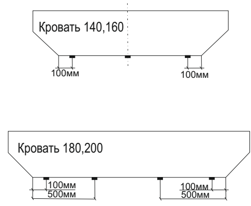
Схема установки подпятников
