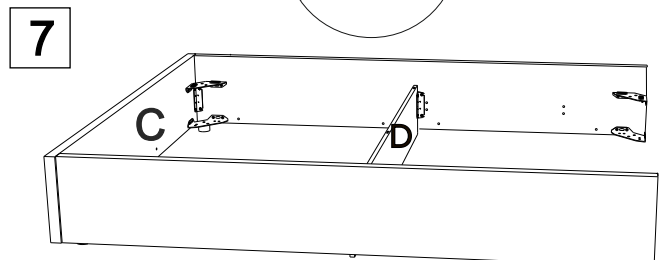
Схема установки подпятников
